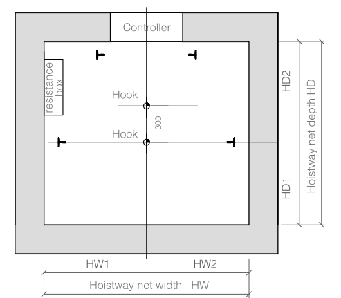
HOISTING HOOK
